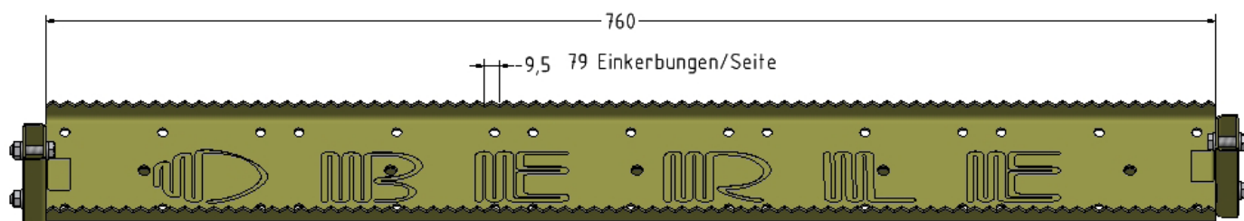
Unterteil PFB 760-9,5-B75
